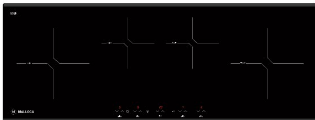
MH-04IR S Bếp kính âm 2 từ, 2 điện Công suất: 0.8kW/1.9kW - 1.2kW - 1.6kW - 2kW Tổng công suất: 6.7kW KT: W930 x D360 x H60mm KT lỗ đá: W895 x D325mm Giá: 32.340.000đ
