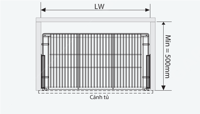
Giá bát đĩa, rổ nan đẹt, cánh mở GD04E Inox 304, bề mặt điện hóa xước mờ
