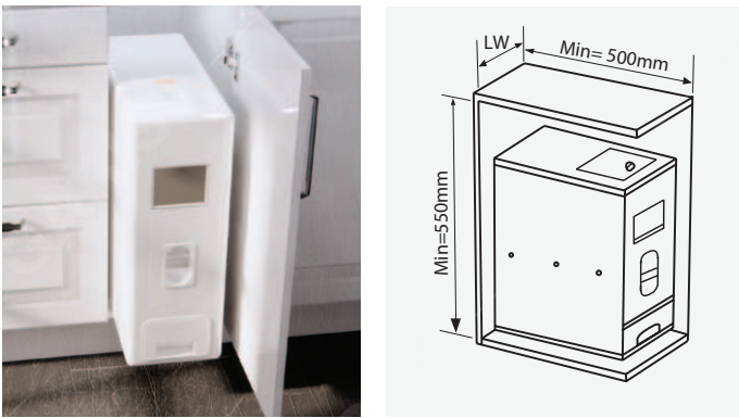
Thùng gạo 15kg, cánh mở, KT mặt cánh 250mm GR02.25 1 khoang, thùng bằng thép sơn tĩnh điện, mặt nhựa ABS
