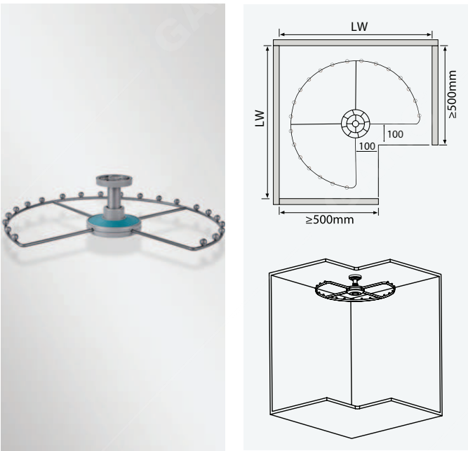
Giá xoay GW32E, treo trần góc tủ quần áo, 1 tầng
