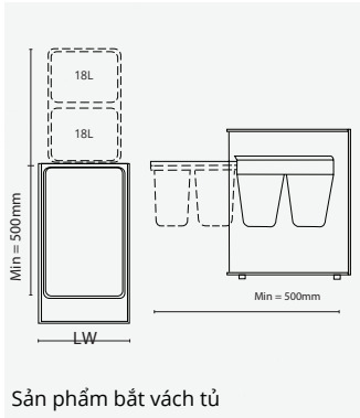
Sản phẩm bắt vách tủ
