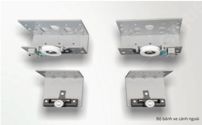
Bộ bánh xe cánh ngoài
