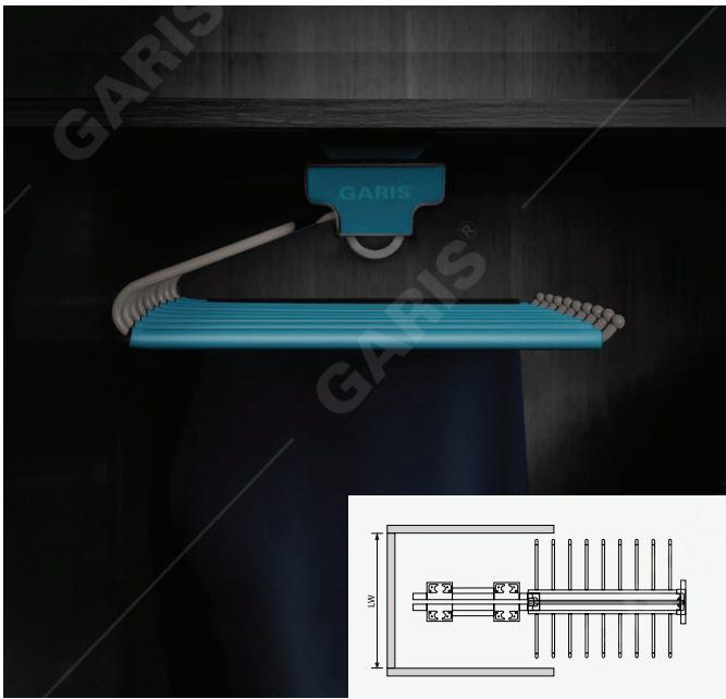
Giá treo quần âu đơn cân GW38E
