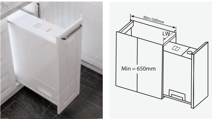
Thùng gạo 15kg, cánh kéo, KT mặt cánh 200mm GR01.20 1 khoang, thùng bằng thép sơn tĩnh điện, mặt nhựa ABS
